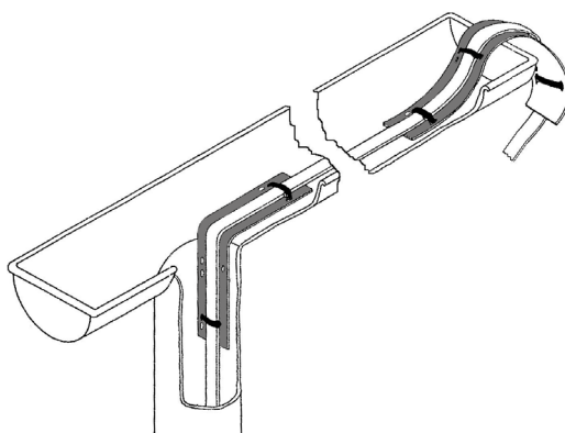
40049014 – Schützt das Heizkabel beim Übergang von der Dachrinne zum Fallrohr
