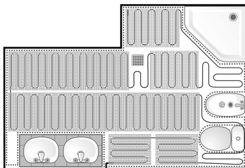
Рис. 1. Чертеж пола
