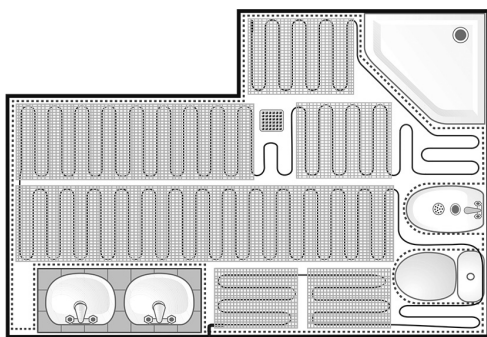
Fig. 1. Golvvritning
